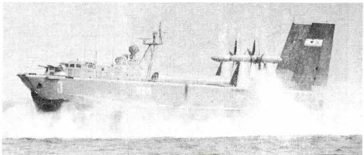
Sovjetisk AIST-klasse luftpude fartøj. 45 x 18 m. DPL: 220 t. Ca. 250 kvm lasteflade
